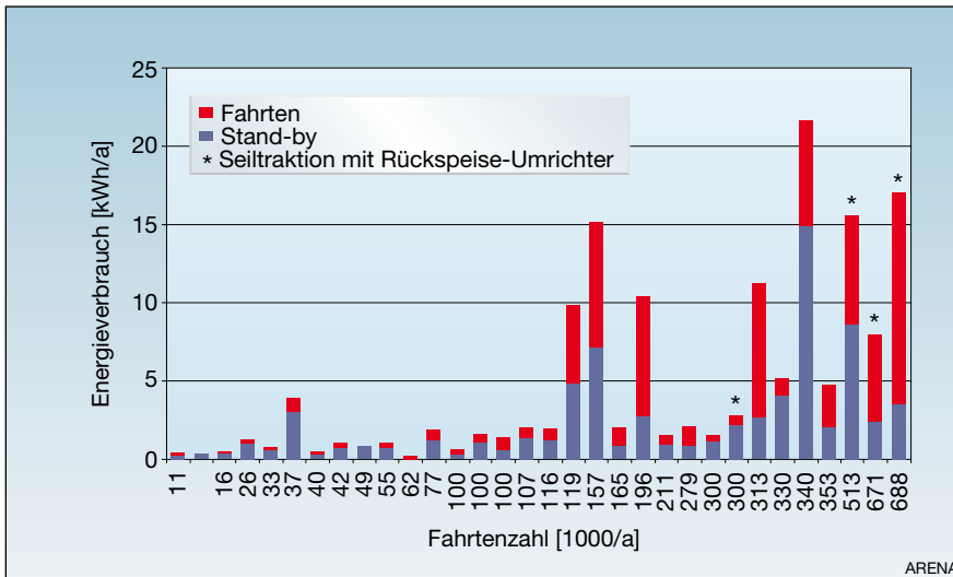
Bild 4 Stand-by- und Fahrten-Energieverbrauch der Aufzüge nach Fahrtzahl
